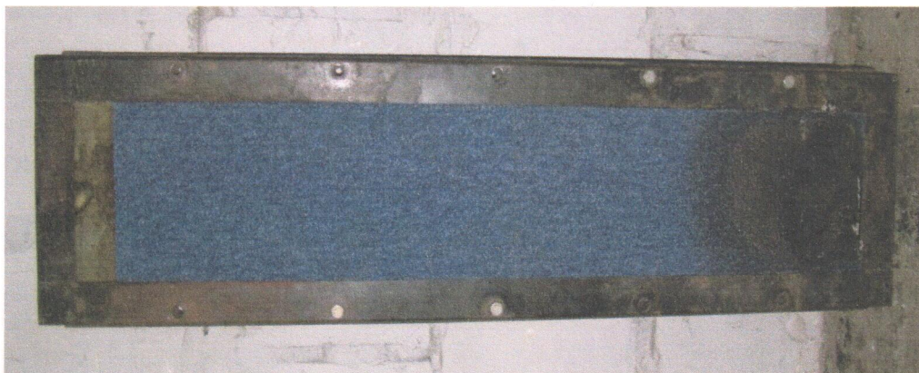
Рисунок 1 - Характерний вигляд зразка килимової плитки для підлоги колекції TESSERA, виробництва «Forbo Flooring UK Ltd.» (Великобританія), після випробувань з визначення групи поширення полум'я згідно з ДСТУ Б В.2.7-70-98.
